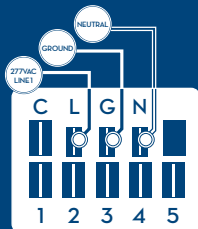
277VAC MOTOR
